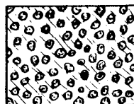
Pelsparite (Ip)
